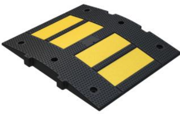
Reductor de Velocidad RE-5 Sección central 505x606x50 mm RE-5-50X60
