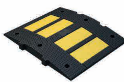
Reductor de Velocidad RE-5 Sección central 505×606×50 mm RE-5-50X60
