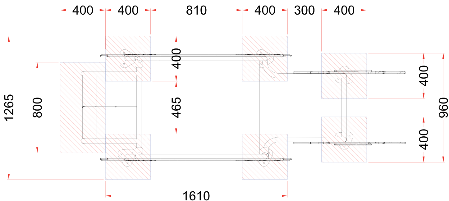
PLANTA CIMENTACION
