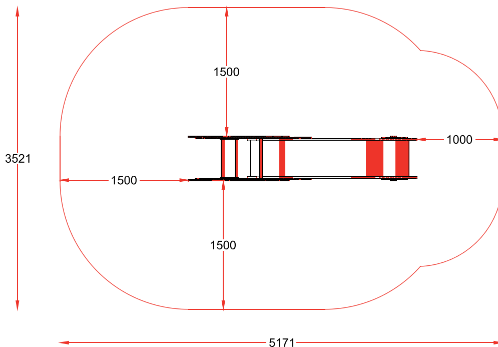
PLANTA CIMENTACION
