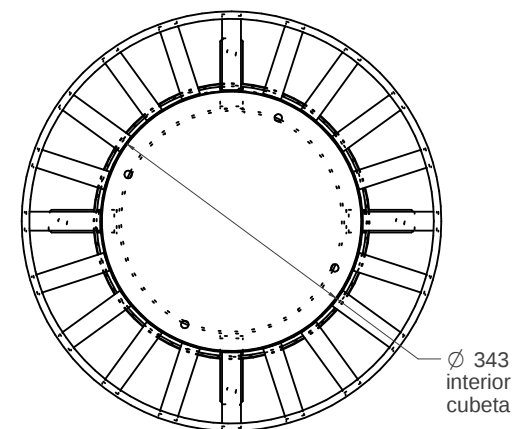
VISTA EN PLANTA 1:10
