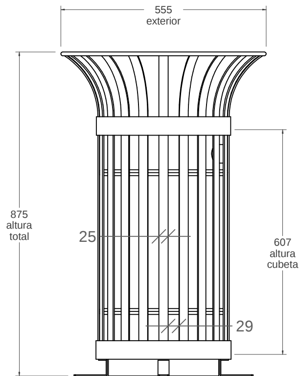
VISTA ALZADO 1:10
