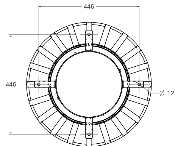
VISTA INFERIOR 1:10
