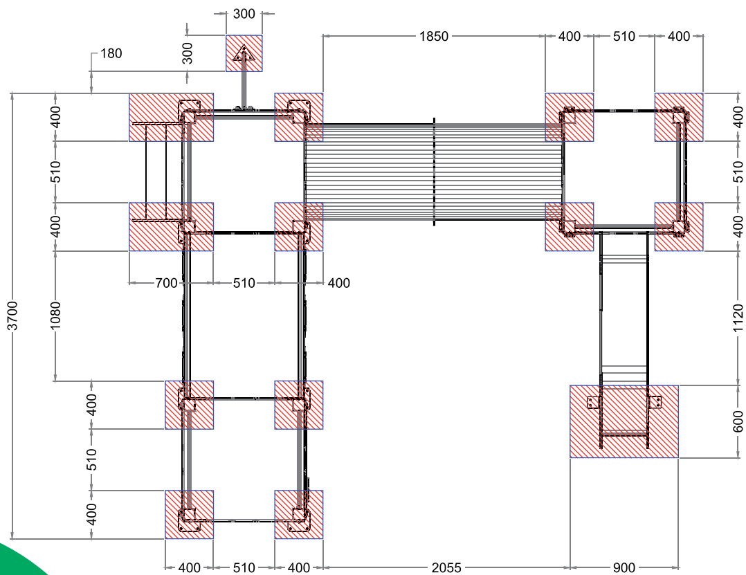
PLANTA CIMENTACION
