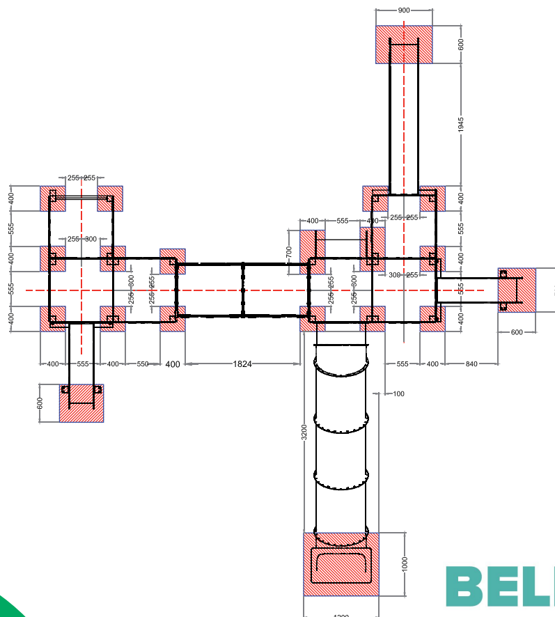
PLANTA CIMENTACION
