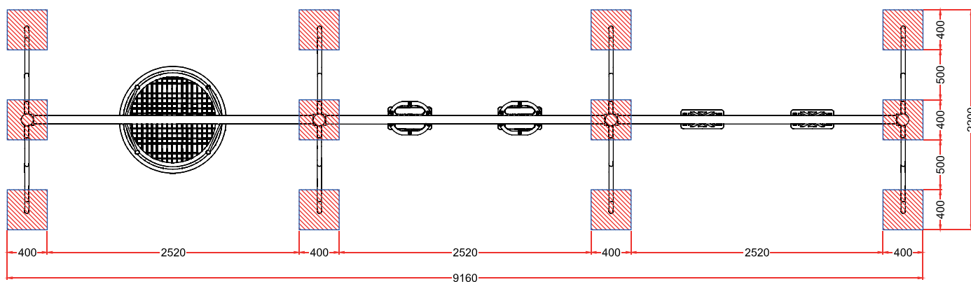
PLANTA CIMENTACION
