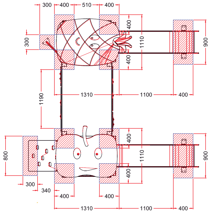
PLANTA CIMENTACION
