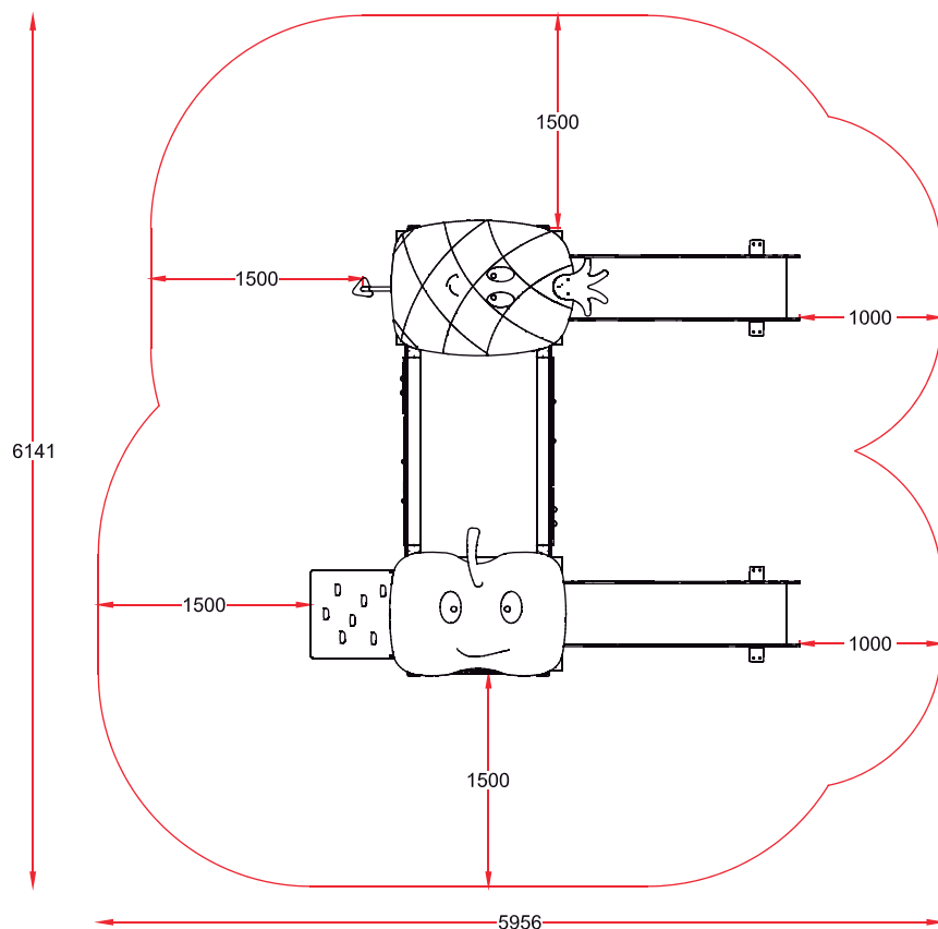
PLANTA
