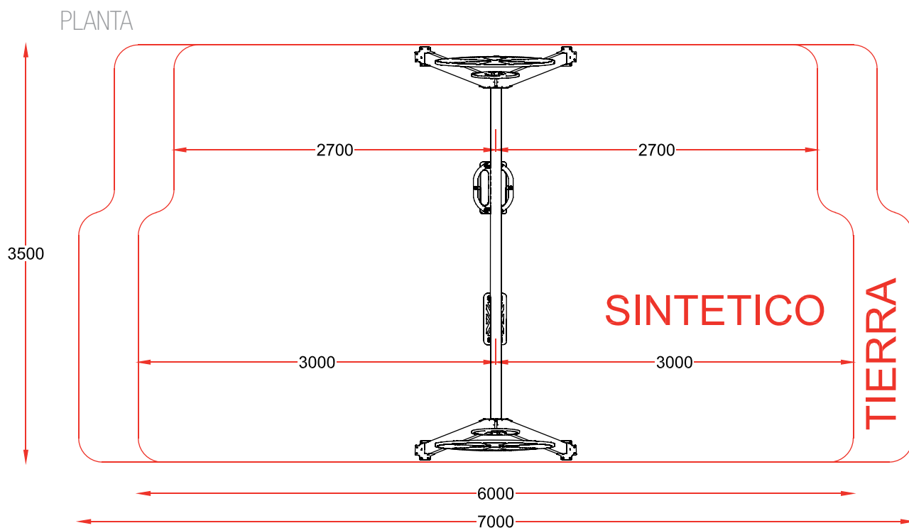
PLANTA CIMENTACION
