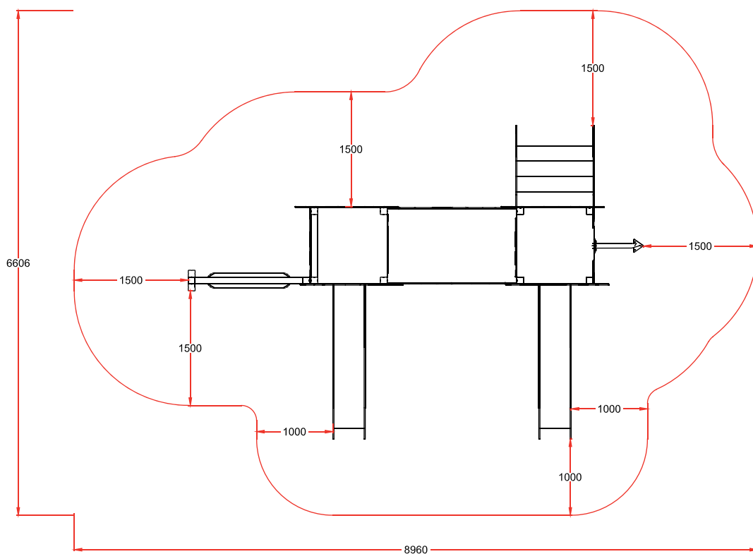
PLANTA CIMENTACION
