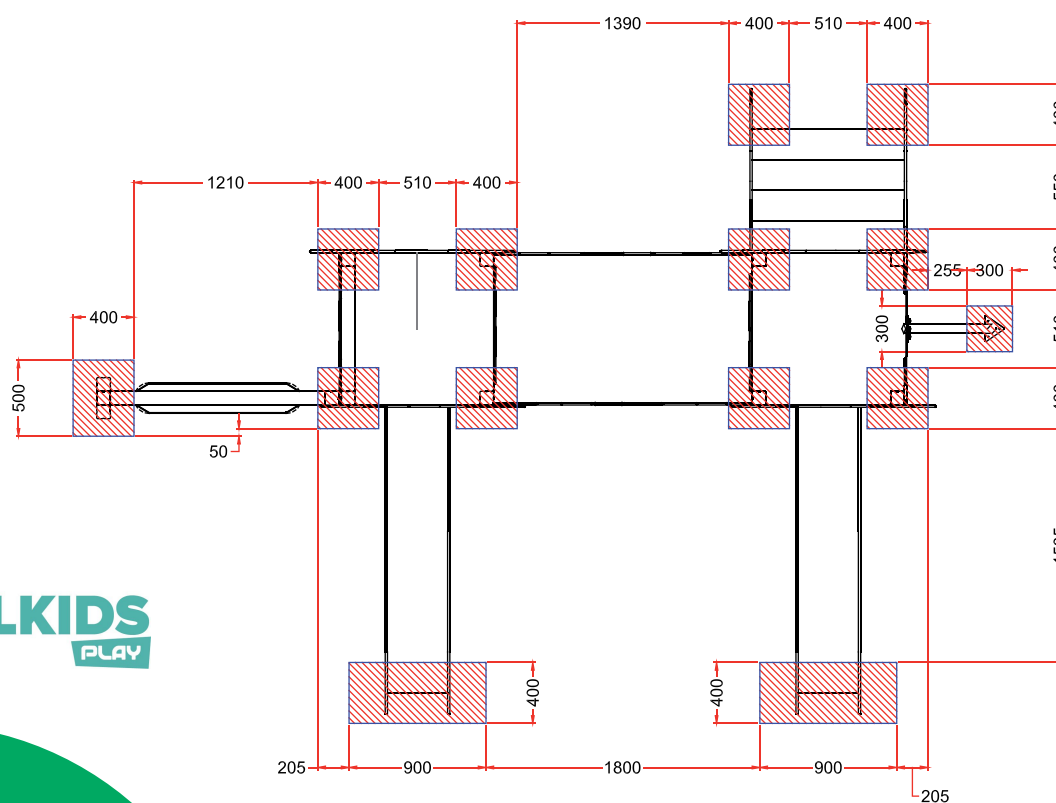
PLANTA CIMENTACION
