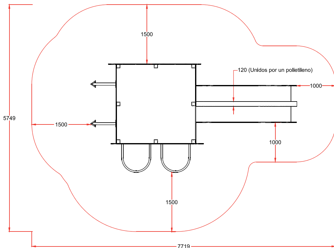
PLANTA CIMENTACION
