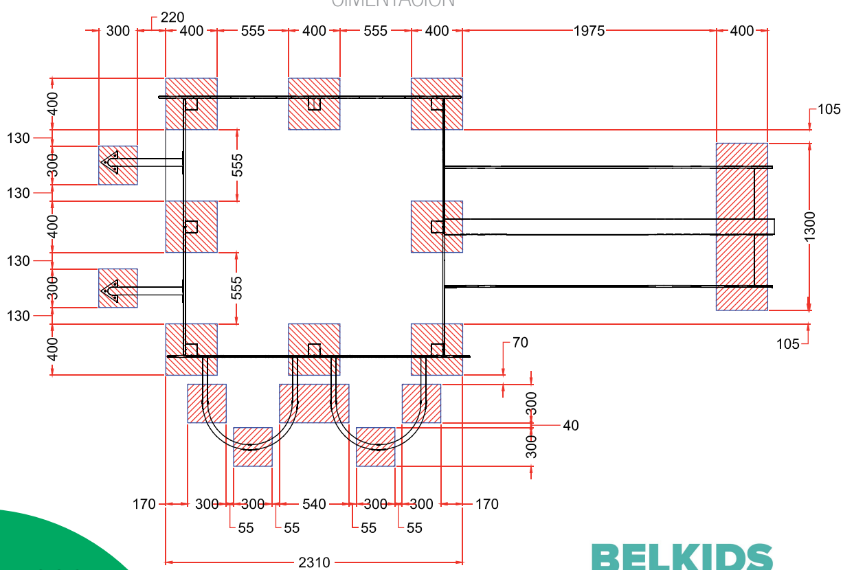
PLANTA CIMENTACION
