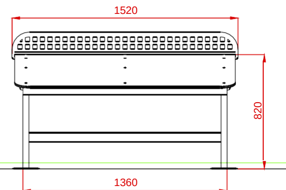
PERFIL
