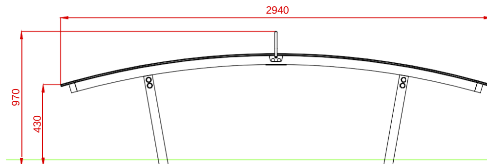
ALZADO
