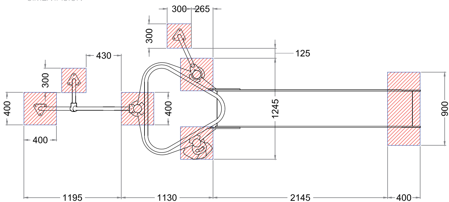
PLANTA CIMENTACION
