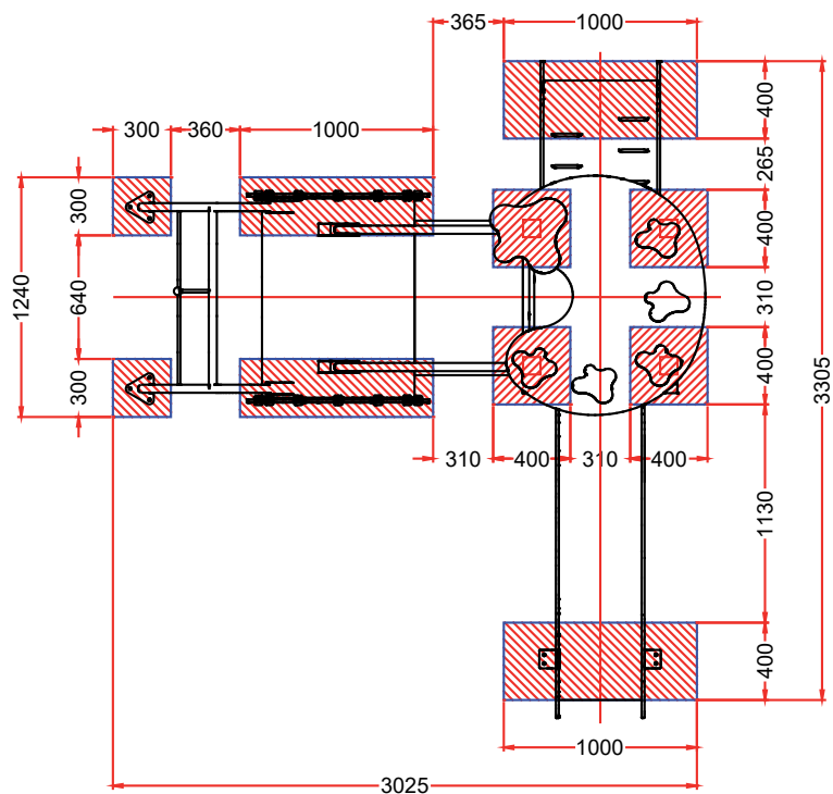
PLANTA CIMENTACION
