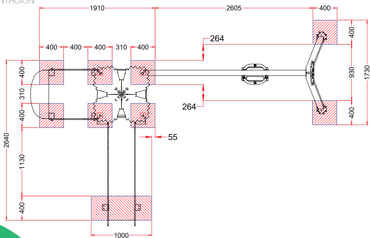
PLANTA CIMENTACION
