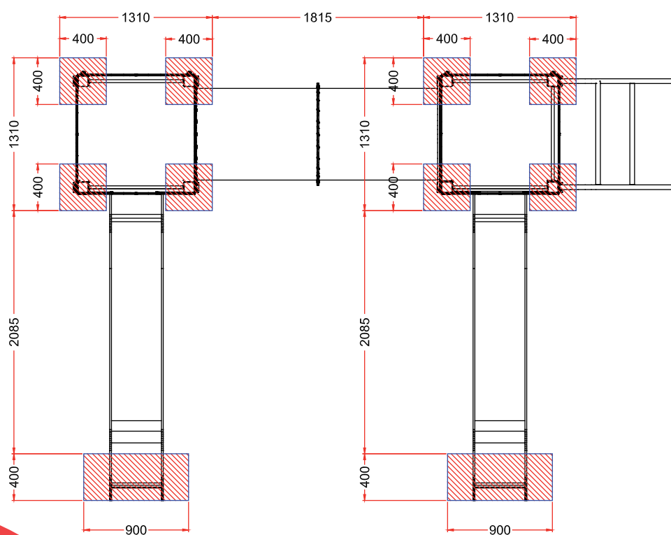
PLANTA CIMENTACION
